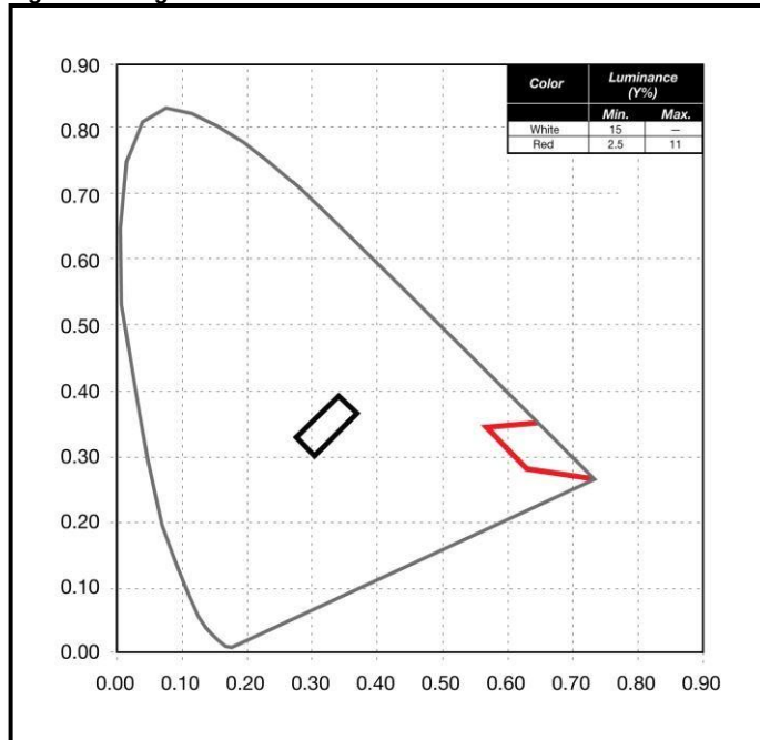
Figura A: Diagrama cromático de la CIE
